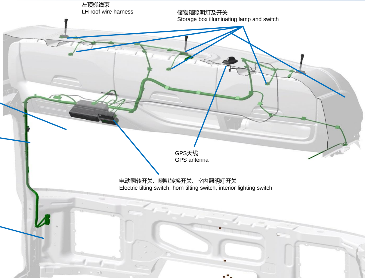
左侧线束接口 LH wire harness interface
